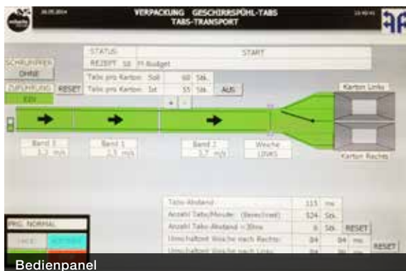
Bedienpanel
