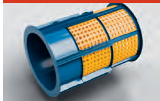
Tamis plat pour cylindre de triage en div. longueurs, élément intérieur
