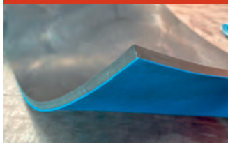
Caoutchouc d'usure avec et sans couche collante 40°/60° shore, 2000 x 10 000 mm H: 6, 8, 10, 15, 20 mm
