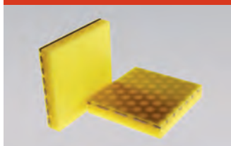
Plaques PU 1000x2000 mm 65°/ 85° Shore Épaisseur: 12, 15, 20 mm avec ou sans tôle perforée
